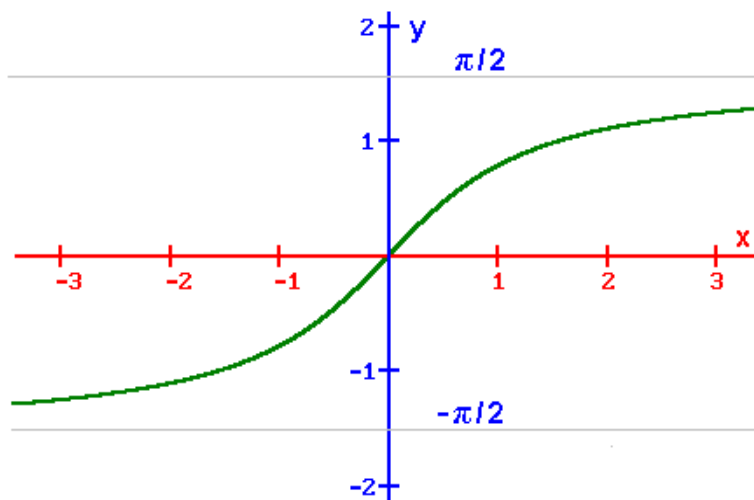
Obrázek 22: Graf funkce arkus tangens, viz http://84.242.77.122/ uc%282ebnice CS/Matematika analiza/Funkce /Elementarni funkce/Goniometrické funkce/atg.GIF
