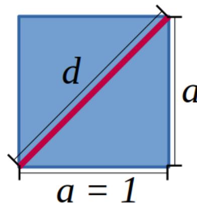
Obrázek 15: Úhlopříčka jednotkového čtverce
