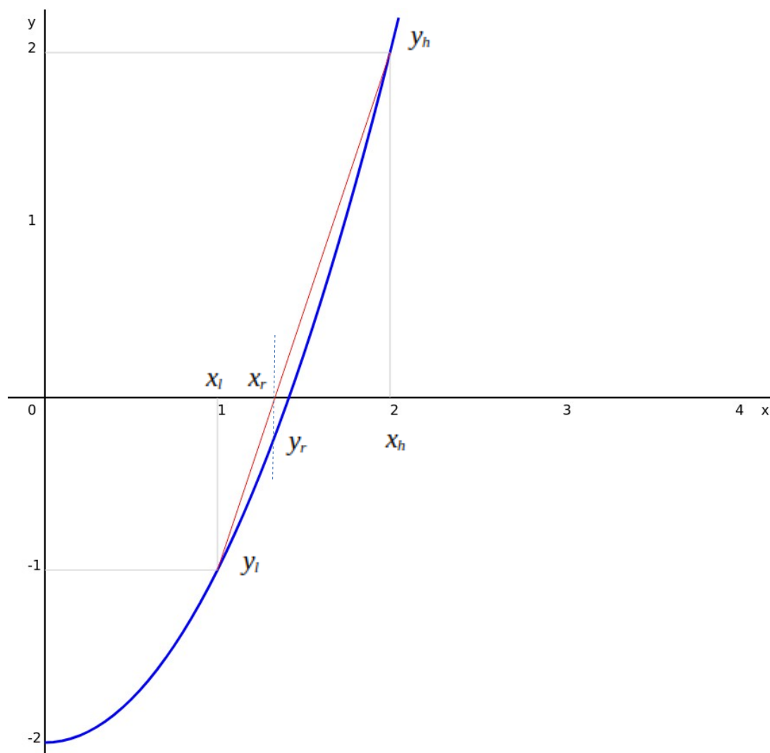
Obrázek 19: Hledání odmocniny metodou sečen, výchozí stav
