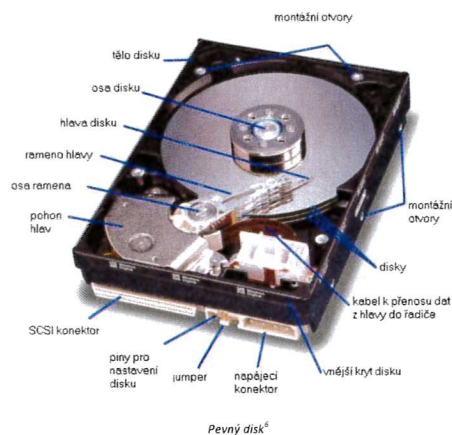
Pevný disk 6
