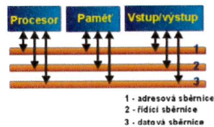
Zobrazení sběrnic
