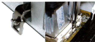
Přítlačnou pružinu na jedné straně zahákneme za plastový úchyt
