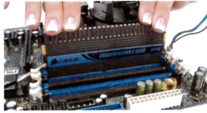
Montáž paměťového modulu
