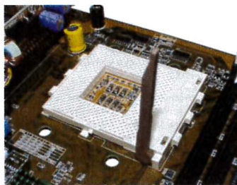
Nadzvednutí páčky
