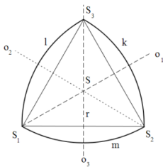
Sférický trojúhelník
